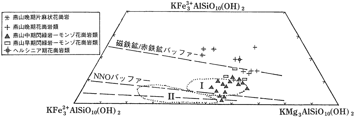
第5図 北京市北方花崗岩類の黒雲母の \text{Fe}^{3+}/\text{Fe}^{2+} 比(郁ほか, 1994). Iは磁鉄鉍花崗岩類の黒雲母の領域, IIはチタン鉄鉍系花崗岩類の黒雲母の領域.
