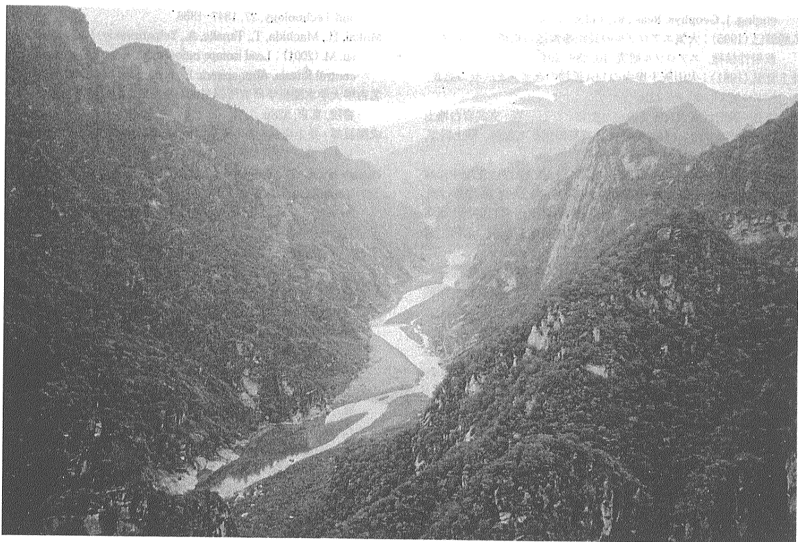
写真1 燕山山地は花崗岩類が谷に刻まれ急崖を造る南画の世界である. そこは近年著しい経済発展をへて2008年にはオリンピックも開かれる北京から, 車で1時間余りの距離である. 東裕村にて.
