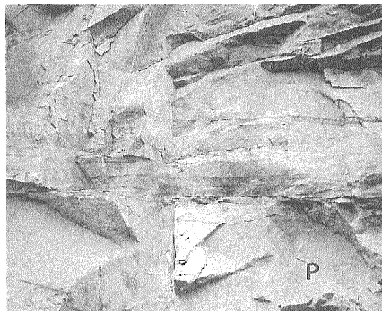
写真10 黒雲母花崗岩中の片状構造。ここでもシュリーレンとペグマタイト岩床が貫入方向と平行に破碎している。最末期にはそれと直交するペグマタイト細脈(P)も晶出。四合堂入口付近。
