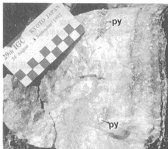
写真15 崎峰茶金山の石英脈鉍石。含金黄鉄鉍(py)が盤際に平行に配列。
