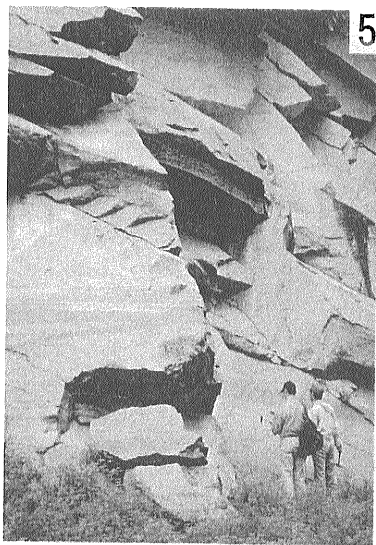
写真5-7 水平方向の縞状構造を持つ燕山期の黒雲母花崗岩類:雲蒙山北縁部. 5 遠景, 6 中景:黒雲母シュリーレンと珪長質岩床が同じ方向の破碎作用を受ける. 7 同クローズアップ:カリ長石は桃色, 一部は斑晶状. コインの直径は23mm.
