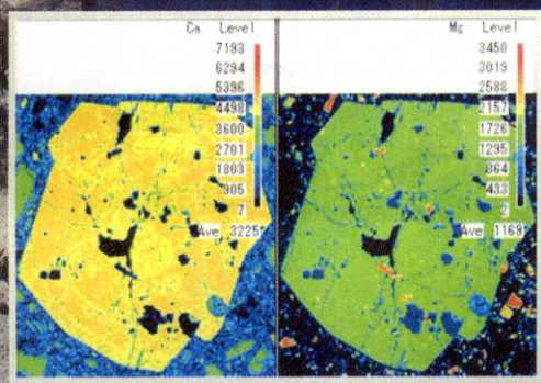
輝石の元素マッピング像
