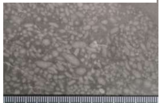
写真2. 金生山産の古生代末の化石 （フズリナ，1目盛は1mm）
