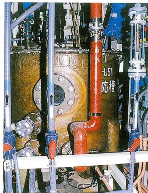
写真3 水銀系廃液分解反応槽
