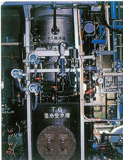
写真6 燃烧排ガス処理用急冷塔
